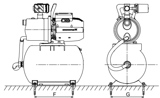
Rys. Fundament dla zestawu podnoszenia ciśnienia JP PT-H
