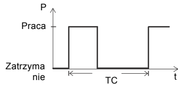
Rys. 10 Tryb pracy S3
