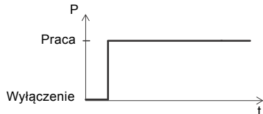
Rys. 11 Tryb pracy S1
